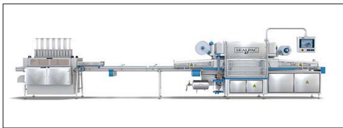
Obr. č. 3: Traysealer SEALPAC A7 a denester AS-LS1200 dokáží zabalit až 100 táček/min (foto SEALPAC)
